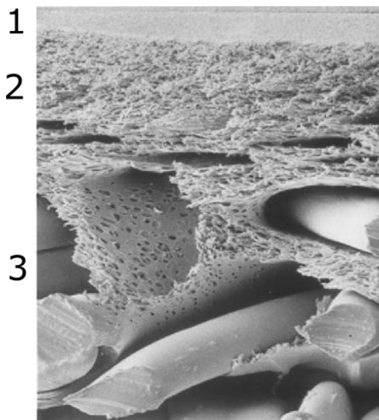
Вид под микроскопом мембранного полотна производства «РМ Нанотех»: 1 – наноструктурированный разделительный слой; 2 – микропористый слой; 3 – нетканое основание
